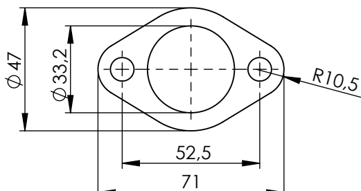
Flange s.s. 43E sp.5mm cod.206308
